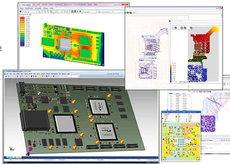
Платформа PADS Professional – маршрут проектирования для инженеров, разрабатывающих сложные печатные платы
