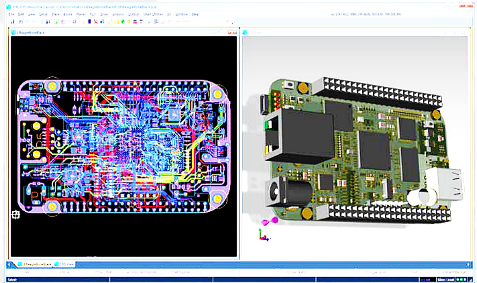
3D-визуализация. Оптимизация и проверка электромеханической конструкции
